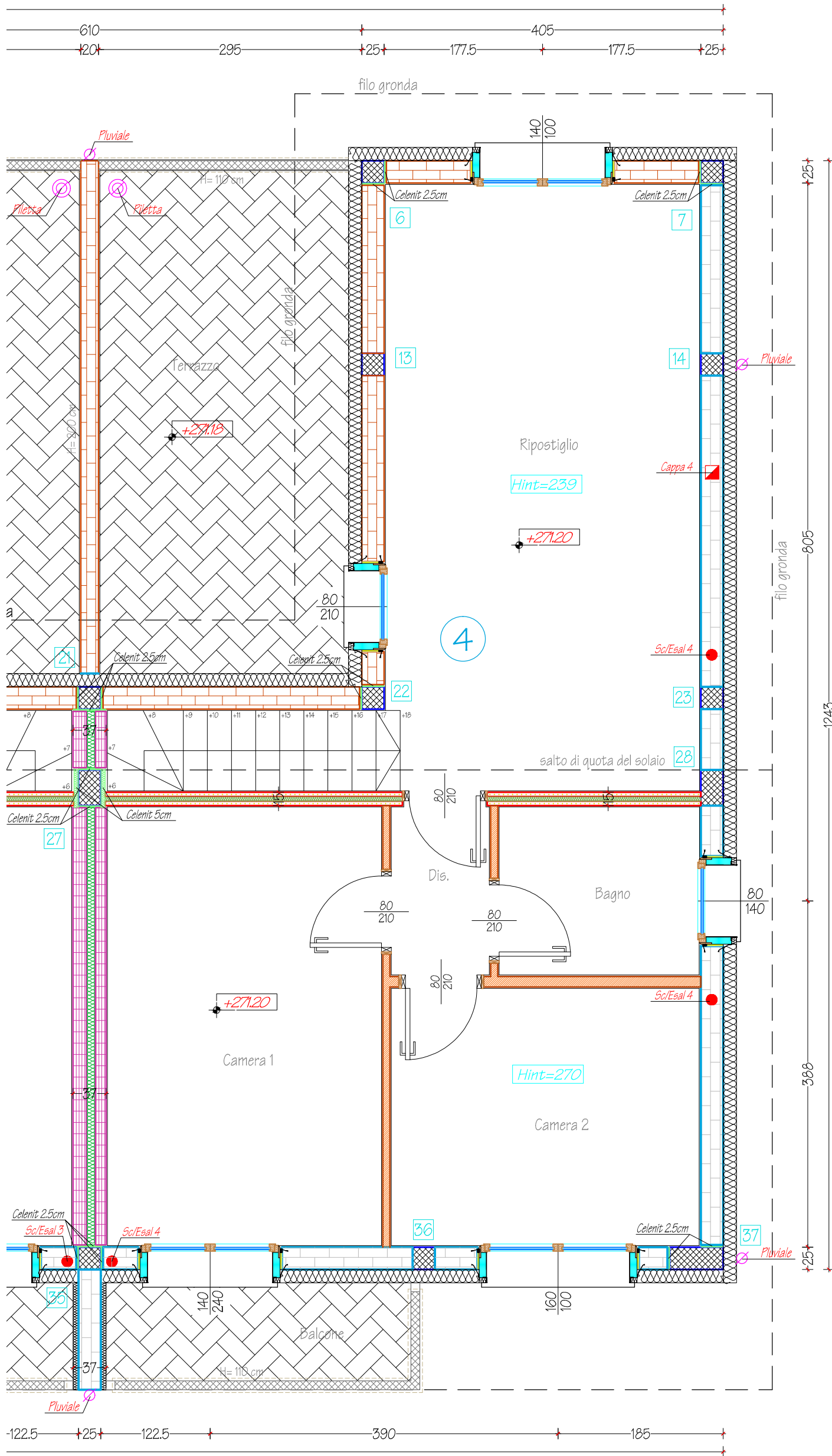
UNITA' 4: PIANTA PIANO PRIMO (Scala 1:50)
