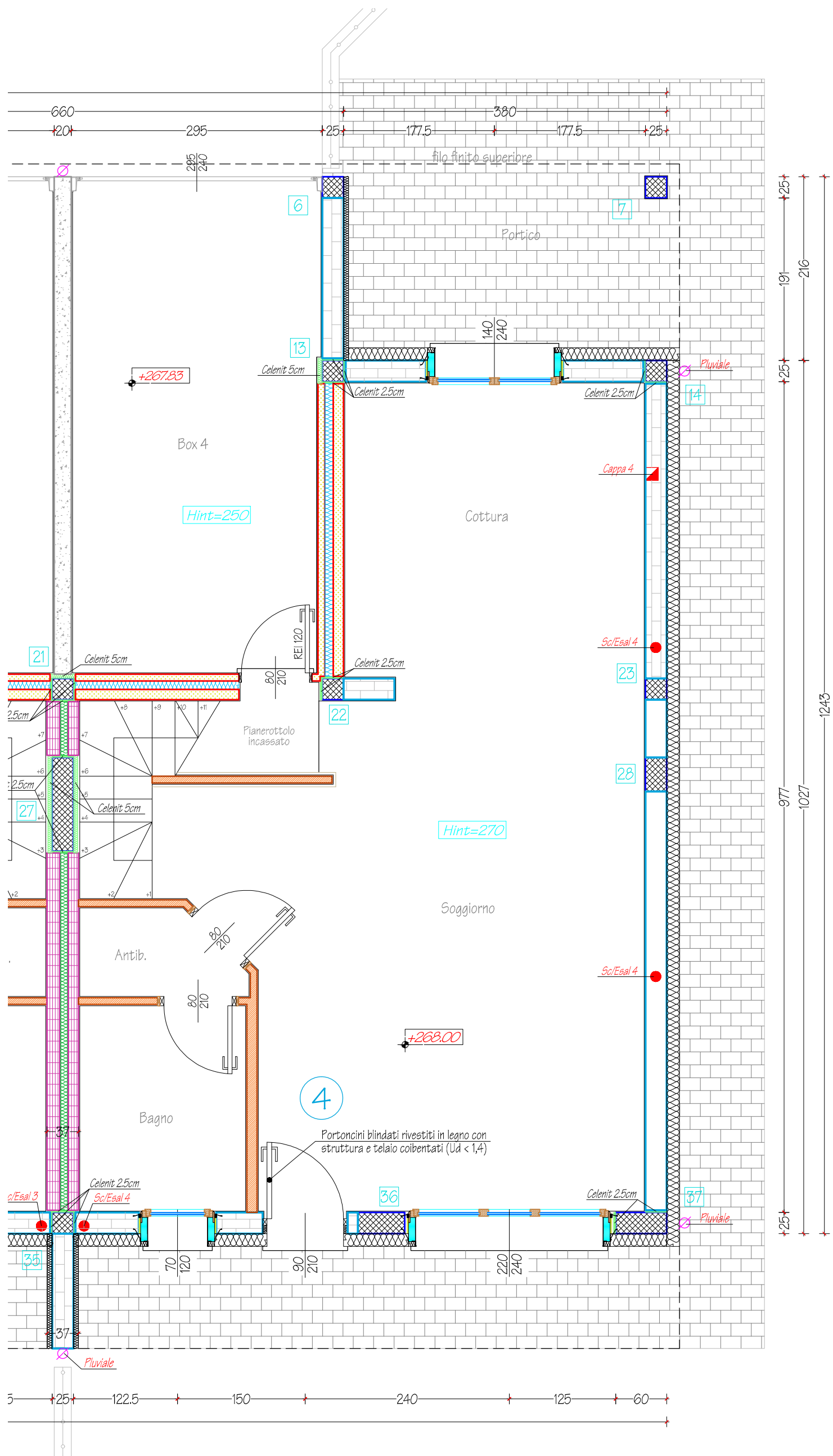
UNITA' 4: PIANTA PIANO TERRA (SCala 1:50)
